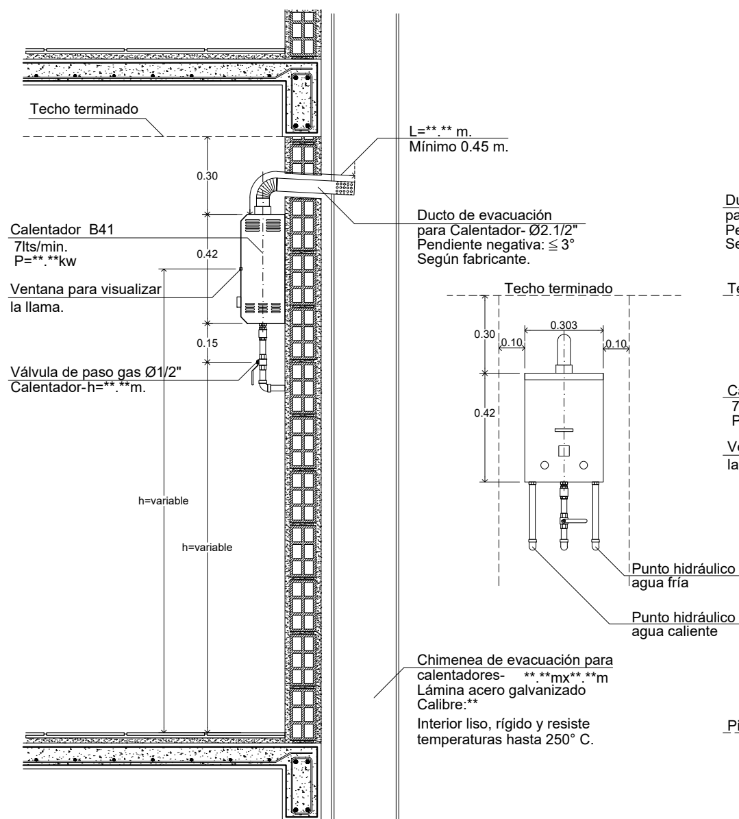
ALZADO
