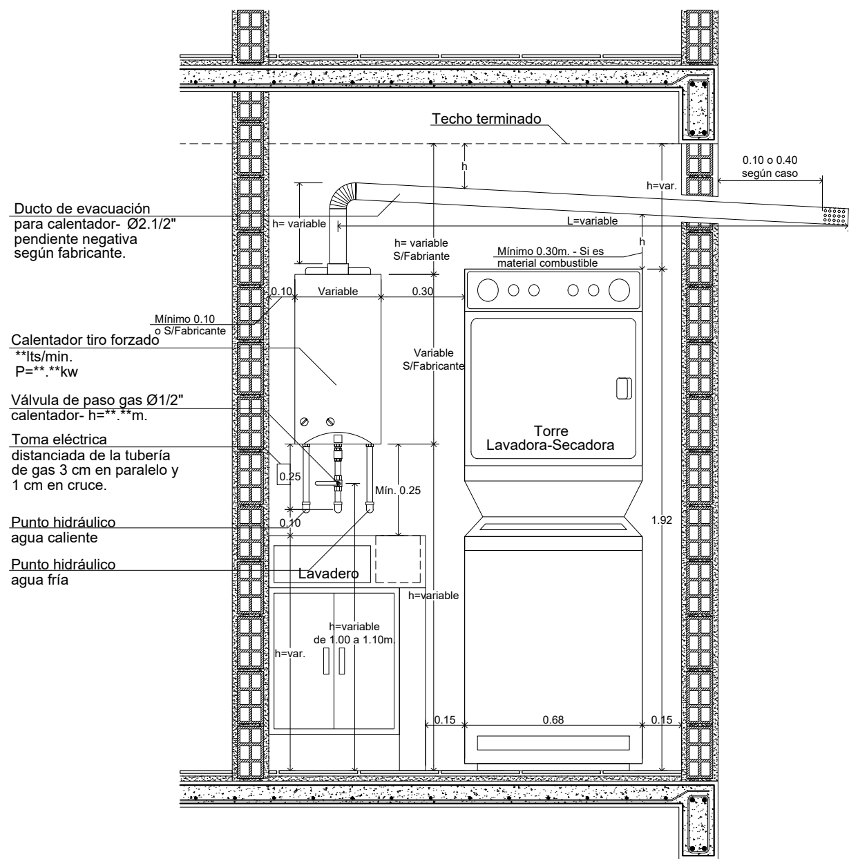
ALZADO
