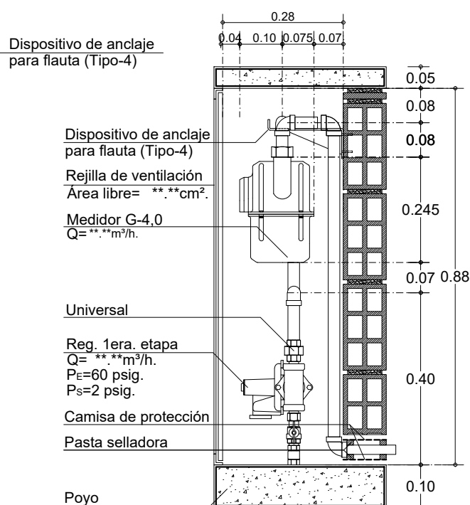
CORTE A-A'
