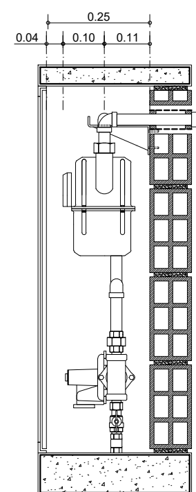
CORTE A-A'
