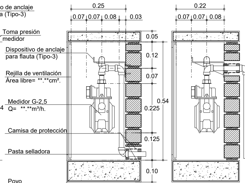
CORTE A-A'
