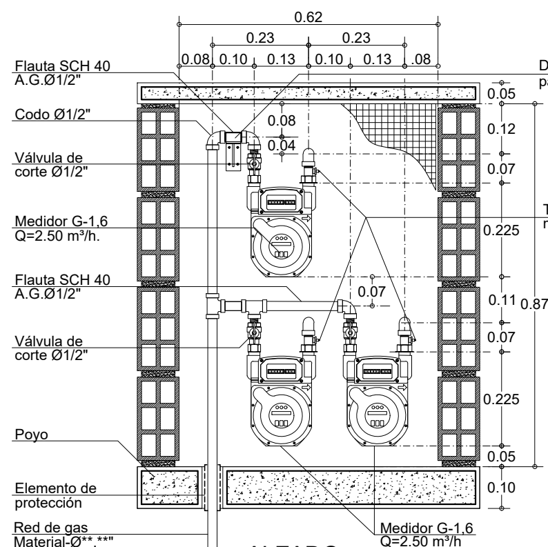
ALZADO
