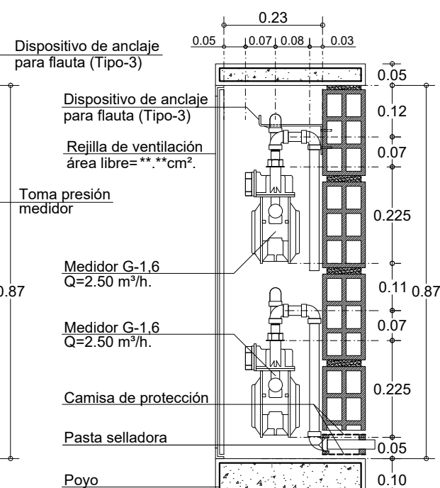
CORTE A-A'
