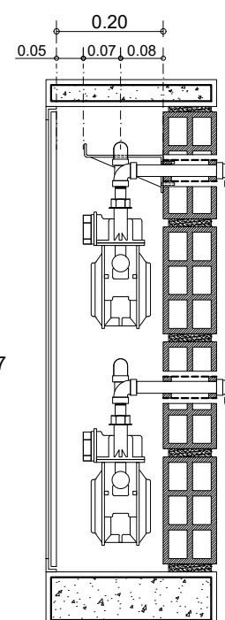
CORTE A-A'
