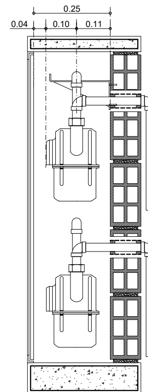
CORTE A-A'
