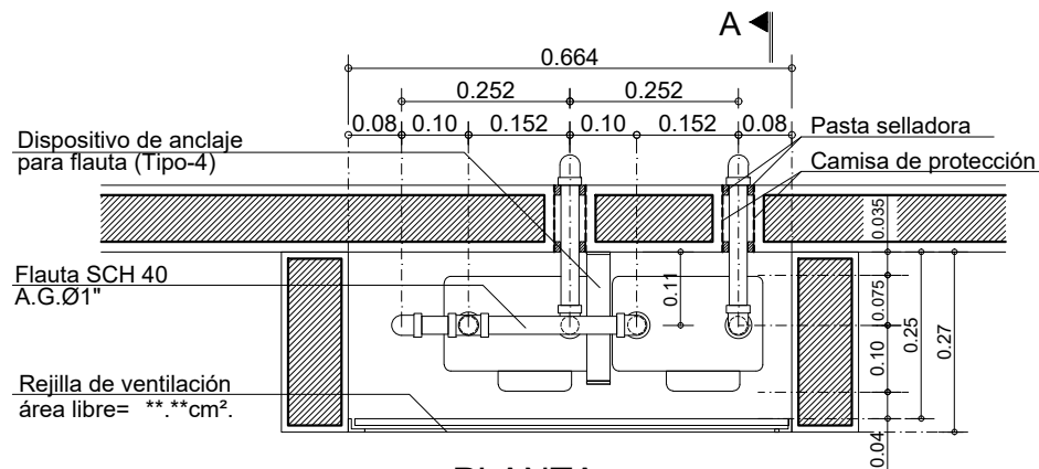
PLANTA
