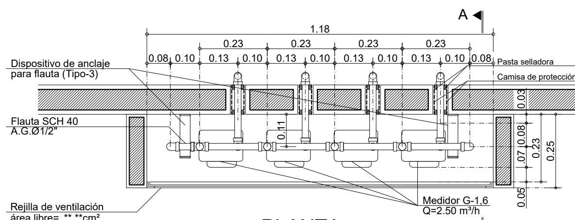
PLANTA
