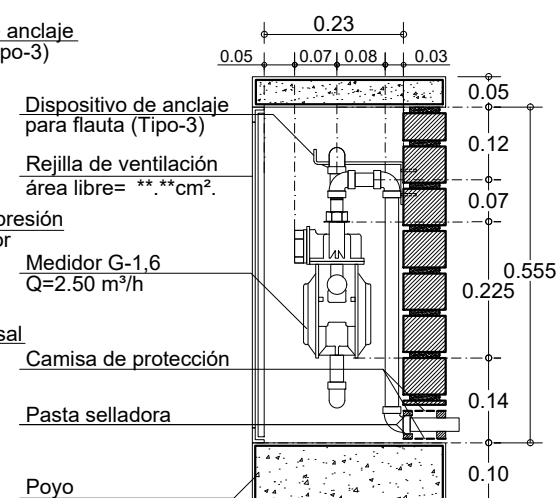
CORTE A-A'
