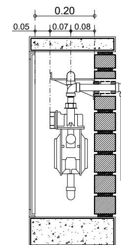
CORTE A-A'
