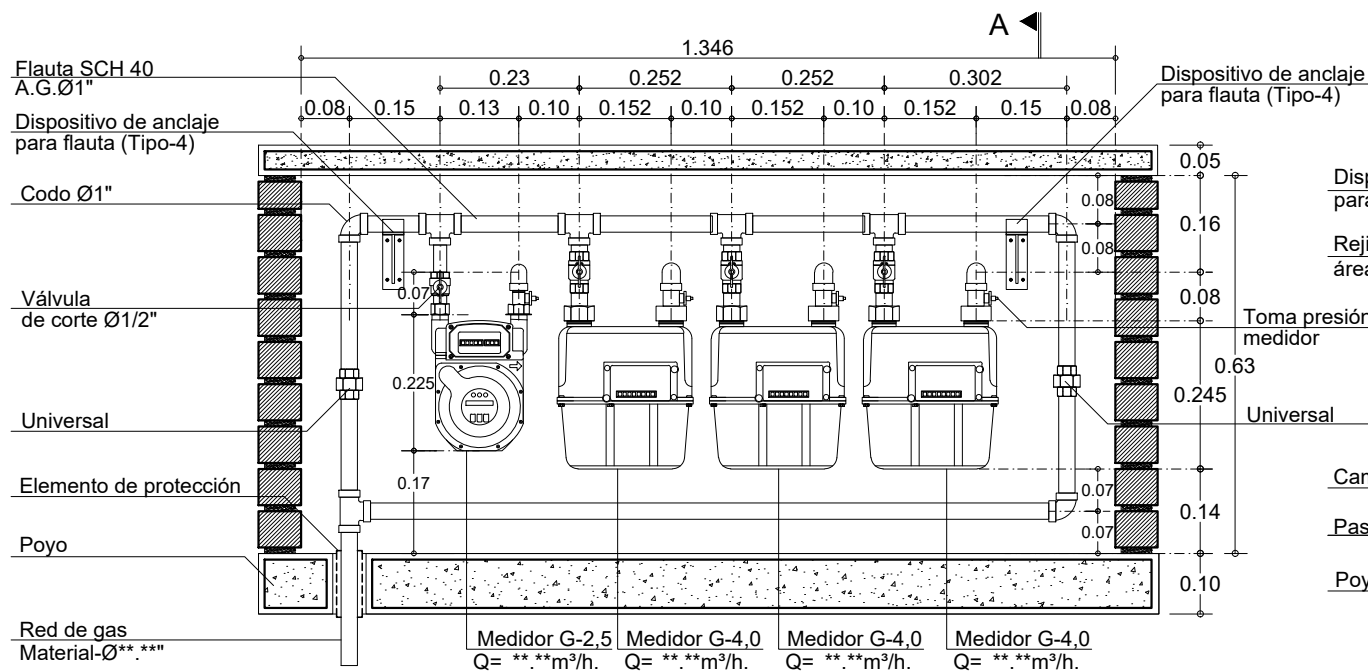
ALZADO
