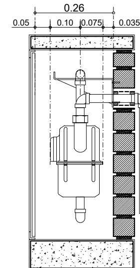
CORTE A-A'
