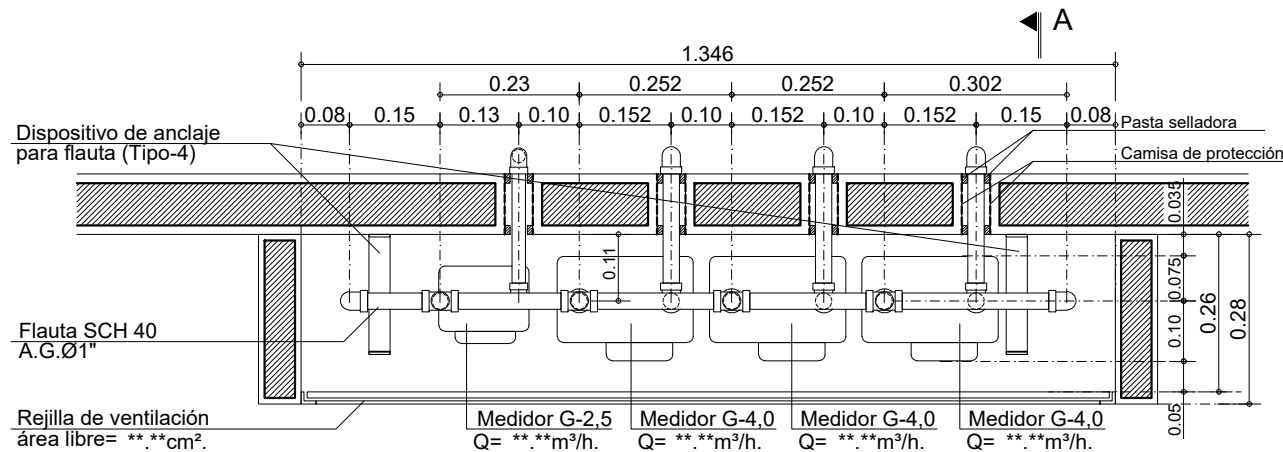
PLANTA
