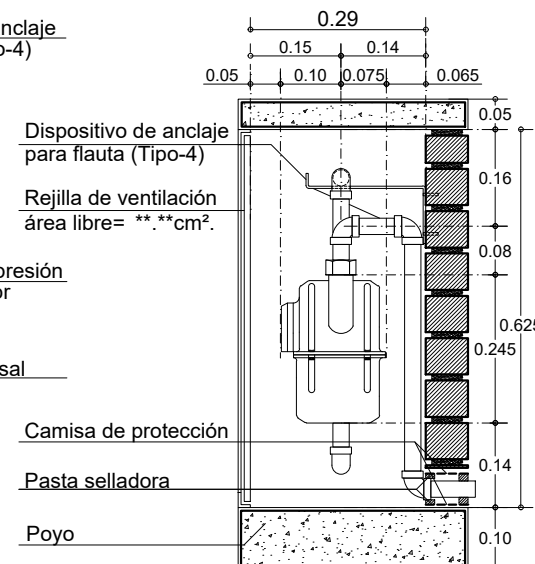
CORTE A-A'
