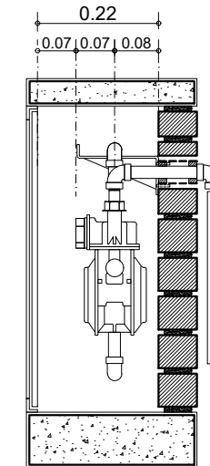
CORTE A-A'
