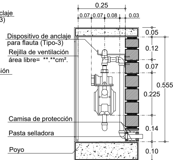
CORTE A-A'
