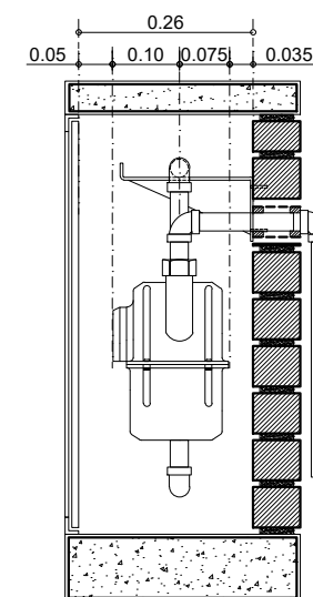
CORTE A-A'
