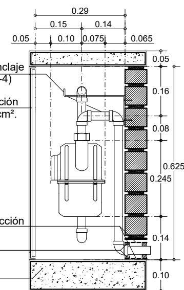
CORTE A-A'
