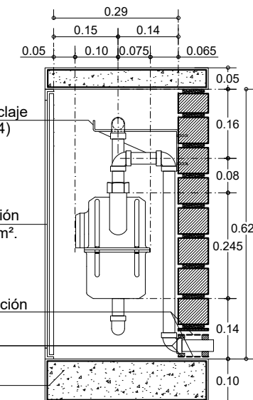
CORTE A-A'
