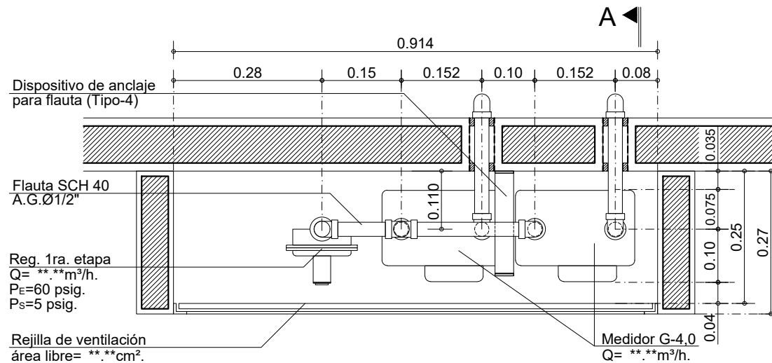
PLANTA
