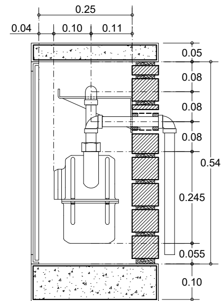
CORTE A-A'
