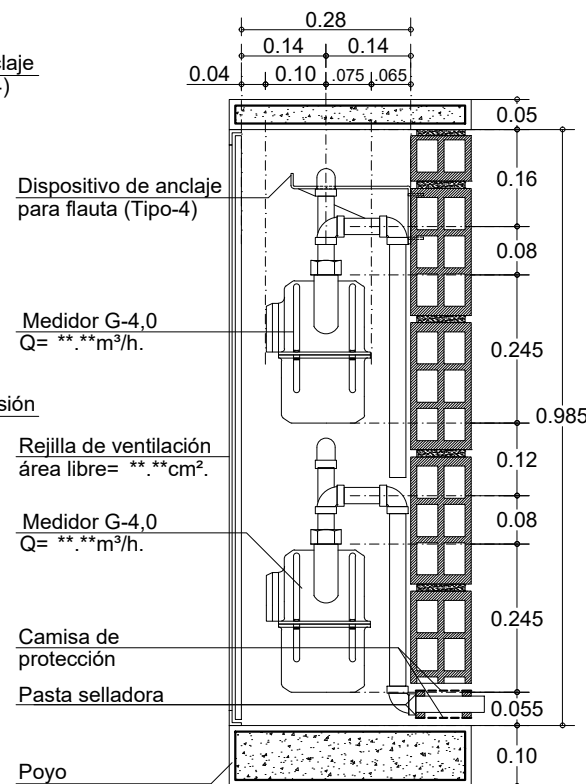
CORTE A-A'
