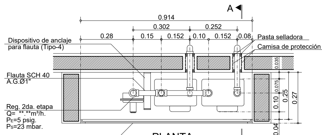
PLANTA
