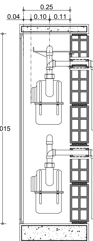
CORTE A-A'
