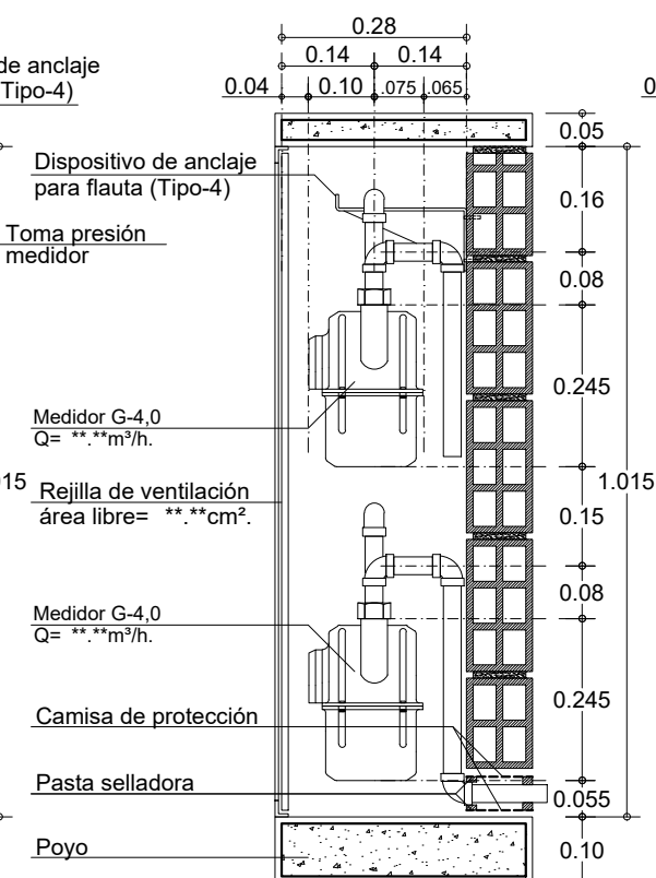
CORTE A-A'
