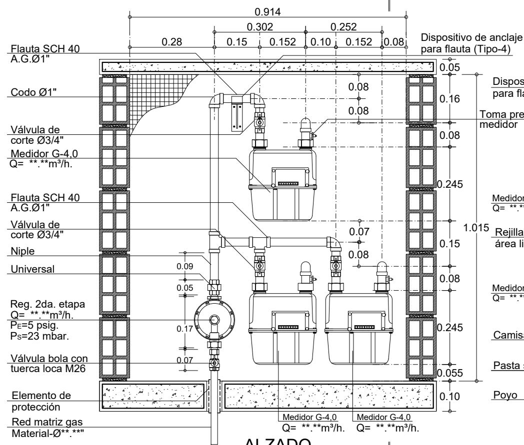
ALZADO
