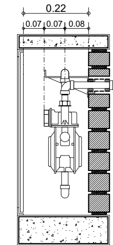
CORTE A-A'
