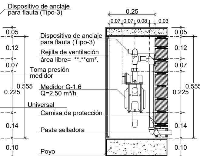
CORTE A-A'
