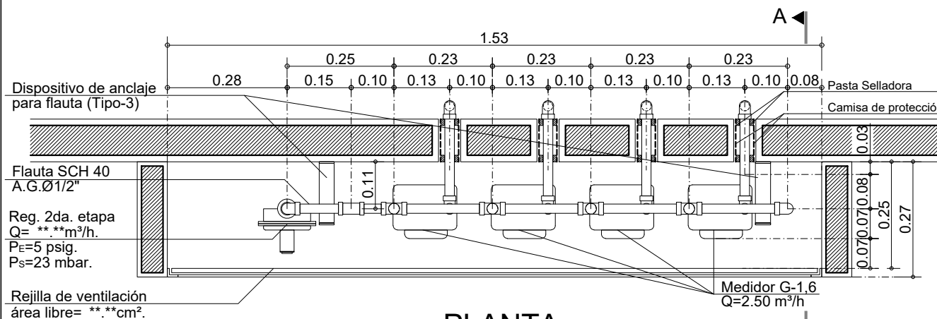
PLANTA
