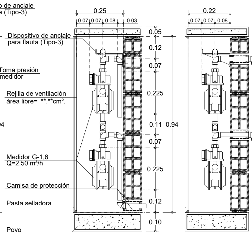
CORTE A-A'
