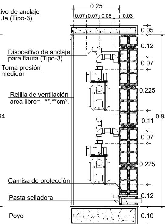
CORTE A-A'
