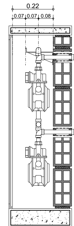
CORTE A-A'
