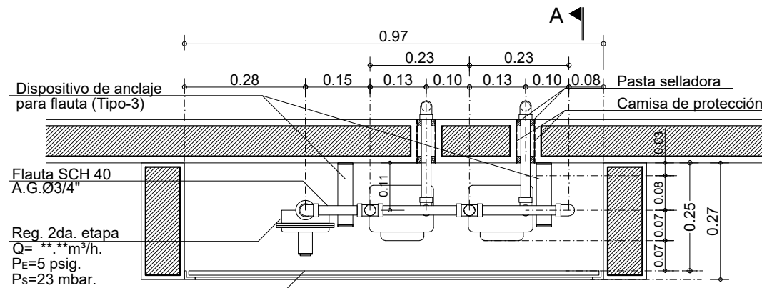
PLANTA
