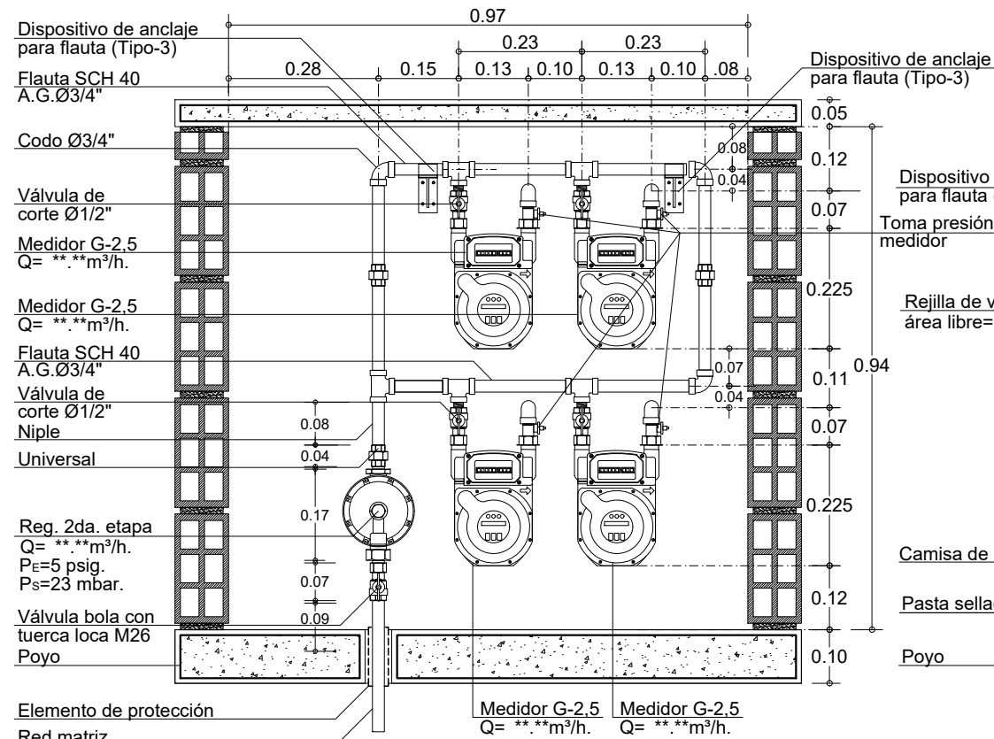
ALZADO
