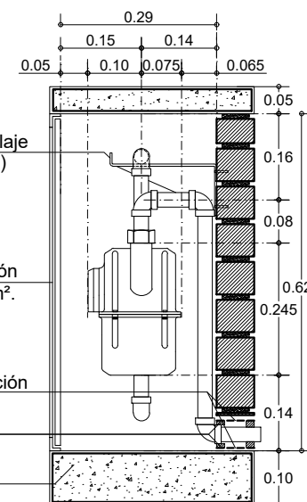
CORTE A-A'
