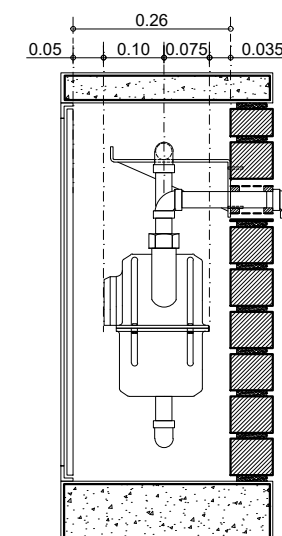
CORTE A-A'
