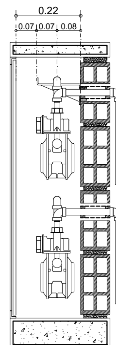
CORTE A-A'
