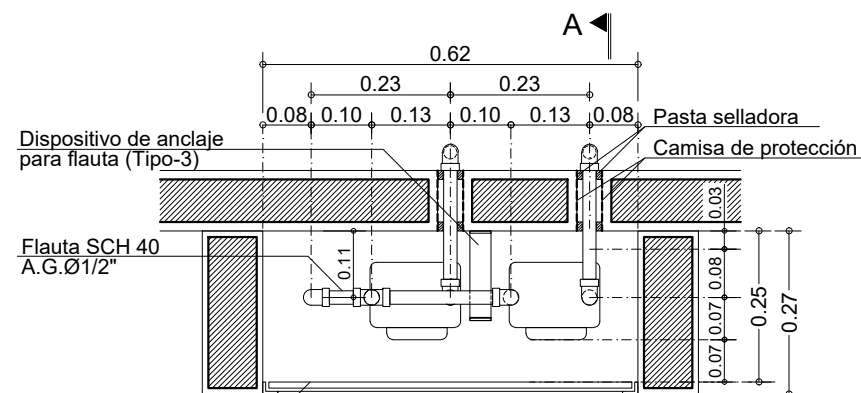
PLANTA
