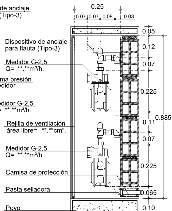
CORTE A-A'
