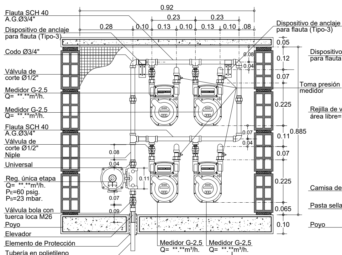
ALZADO
