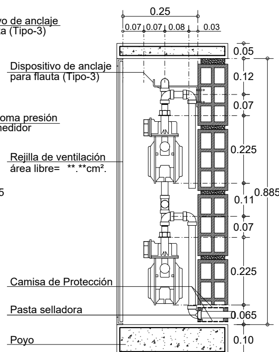
CORTE A-A'
