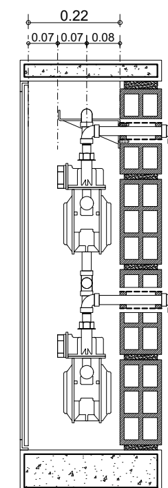
CORTE A-A'
