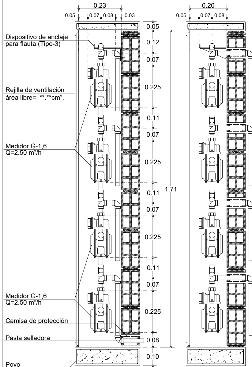
CORTE A-A'
