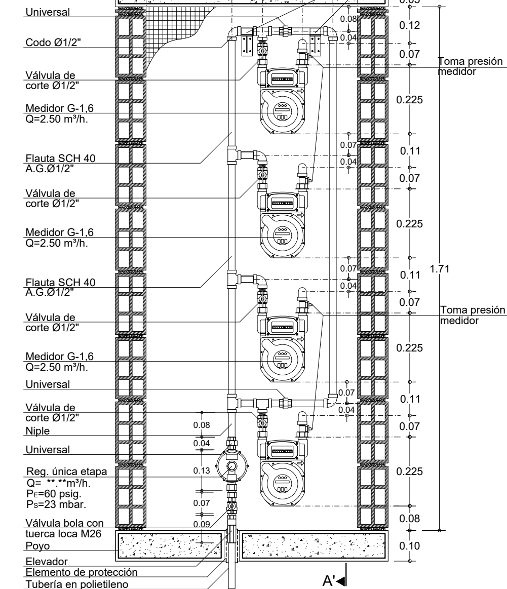
ALZADO
